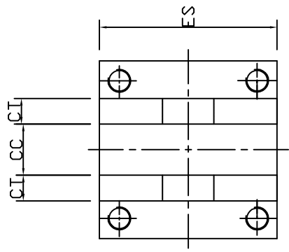
DOUBLE CLEVIS - CL2
